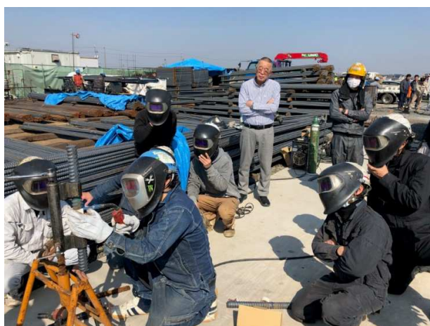
写真三 参加者が横向き溶接を行っています。 SD490 D41ネジ鉄筋を溶接
